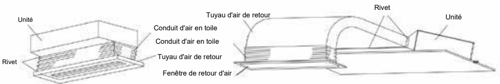
Mode d'installation pour prise d'air par le dessous
